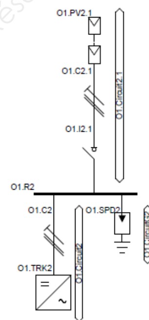
Onduleur 1 entrée B
